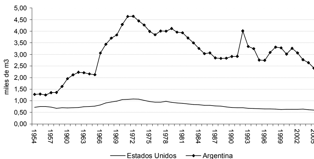
Gráfico 21 – Productividad por pozo en producción efectiva en Argentina y Estados Unidos (1954-2005)
